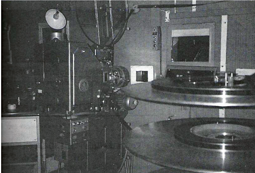
Le projecteur unique et le système à plateaux au premier plan. Le film se déroule depuis le plateau supérieur puis passe dans le projecteur et s'enroule enfin sur le plateau intermédiaire
